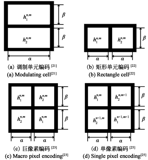
图 3 空间光调制器的双相位编码方式
