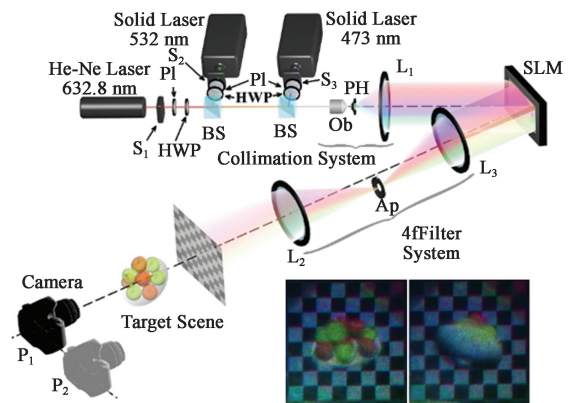
图 8 双相位彩色三维全息显示 [34]
