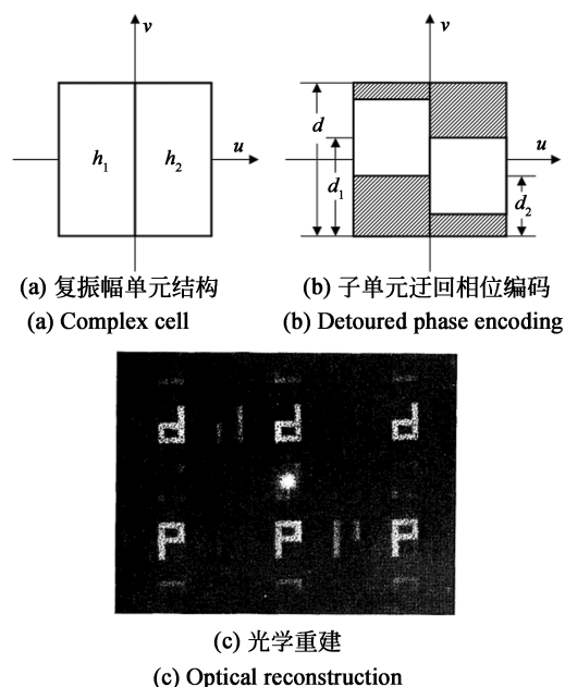
图2 迂回相位编码双相位全息图 [17]
