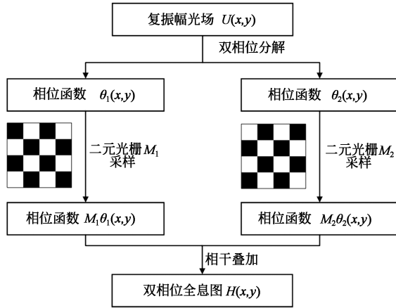
图4 二元光栅采样的双相位图编码流程图 [25]
