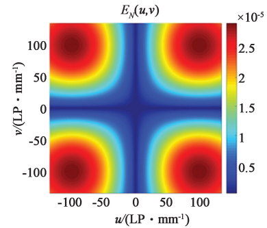
(b) 噪声项外包络函数
