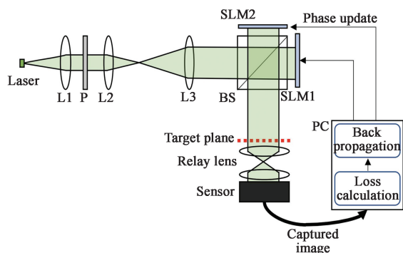
(a) 硬件循环相位干涉系统
