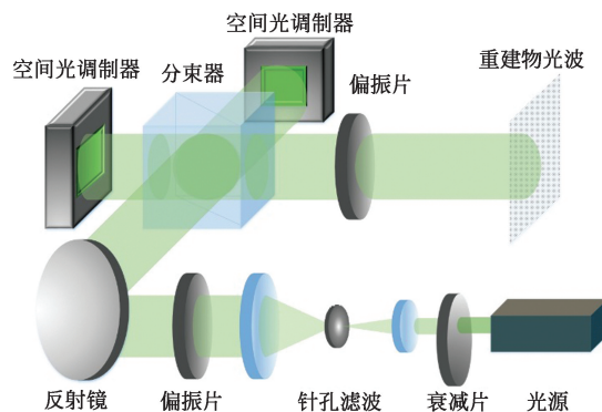
图 12 相位干涉的复振幅全息重建系统
