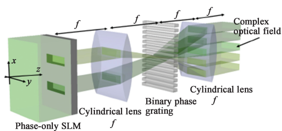
(c) 柱透镜 4f 系统
