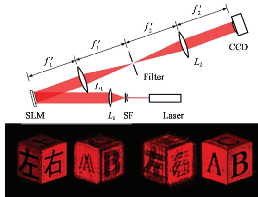
图 7 双相位多层动态全息显示 [33]
