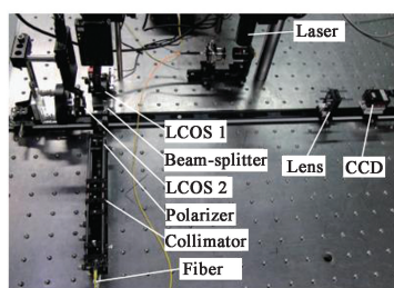
(a) 光学重建系统
