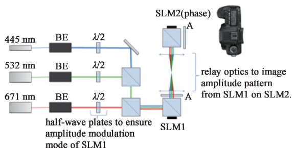
(b) 光学系统
