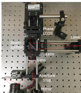
(a) 双相位近眼显示系统
