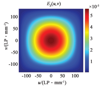
(a) 信号项外包络函数
