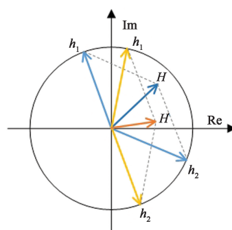
图1 均匀振幅圆内的复振幅分解原理
